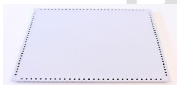
2 x Metallelemente 350 x 350 innen, sichtbare umlaufende Lochreihen
